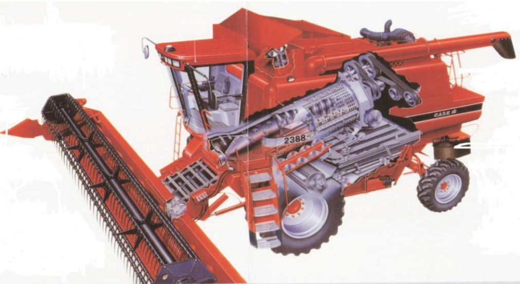
Prostorový řez sklízecí mlátičkou Case axial - flow
