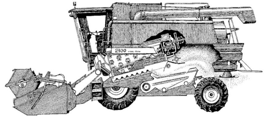
Schéma – prostorový řez stejným strojem
