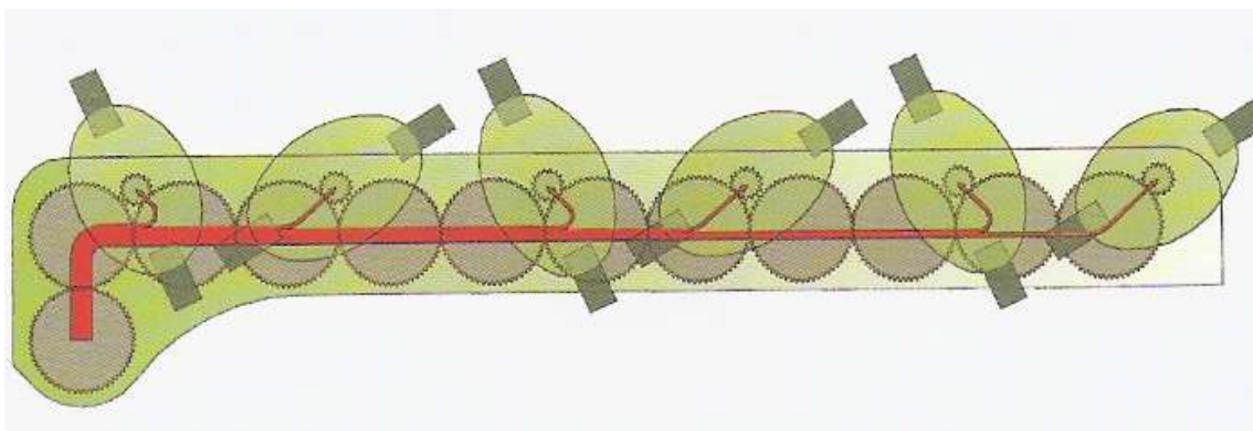
Obr. Schéma převodů žacího ústrojí s plochými rotory
