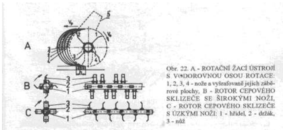
Obr. Žací ústrojí s vodorovnou osou rotace Popis s komentářem pro snadší pochopení:
