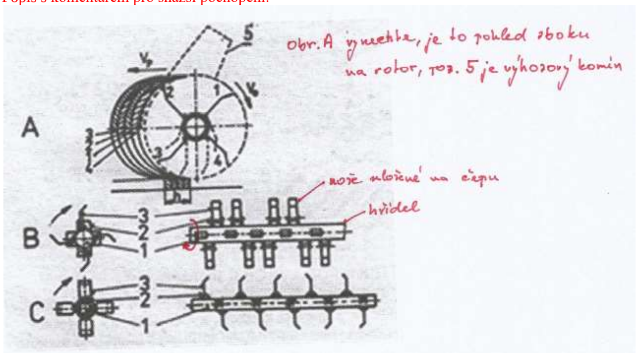
Obr. Žací ústrojí s vodorovnou osou rotace Popis s komentářem pro snadší pochopení:
