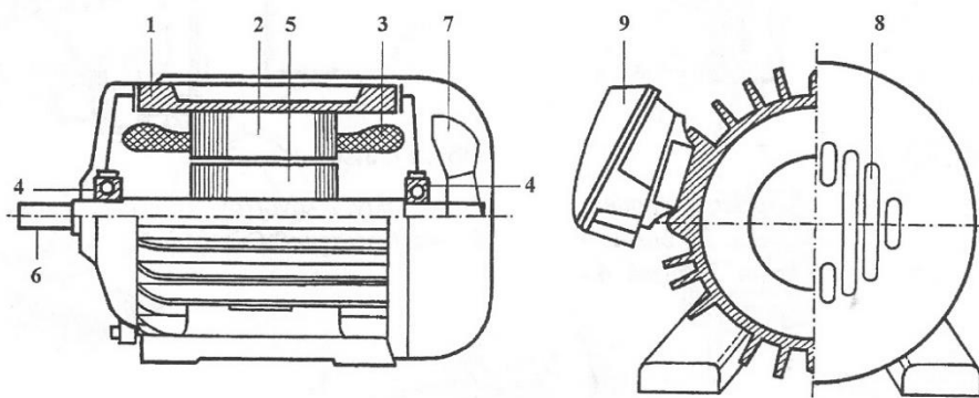
Obr. Trojfázový asynchronní motor s kotvou nakrátko
