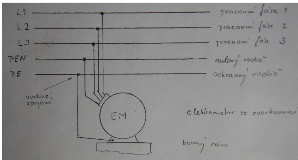
Obr. Ochrana před nebezpečným dotykem
