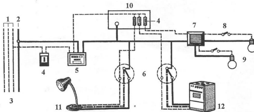
Obr. Příklad domovní instalace bez ochranného vodiče
