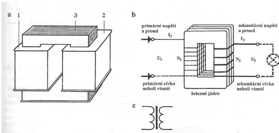
Obr. Transformátor
