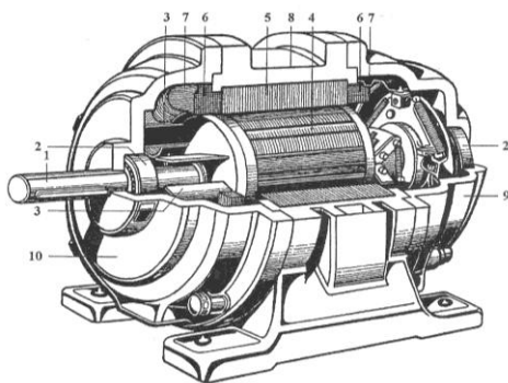
Obr. Jednofázový indukční elektromotor
