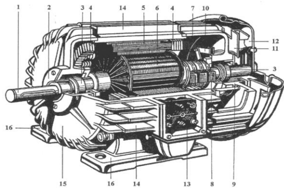
Obr. Trojfázový asynchronní motor s kotvou kroužkovou
