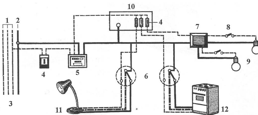
Obr. Příklad domovní instalace v čtyřvodičové soustavě (nyní jen u starších objektů) 1- fázové vodiče, 2- nulový vodič, 3- rozvodná síť, 4- jističe, 5- elektroměr, 6- zásuvka, 7- rozvodná krabice, 8- vypínače, 9- žárovky, 10- rozvodnice, 11- stolní lampa, 12- elektrický sporák
